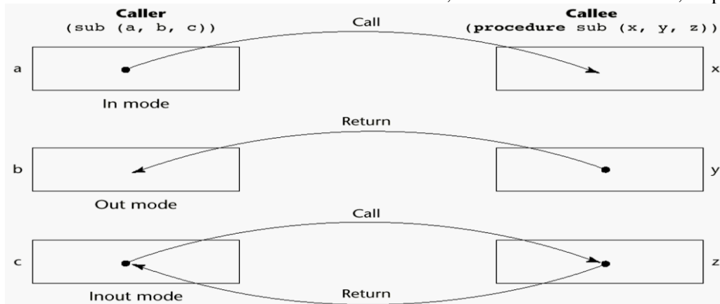
Fig: models of parameter passing
